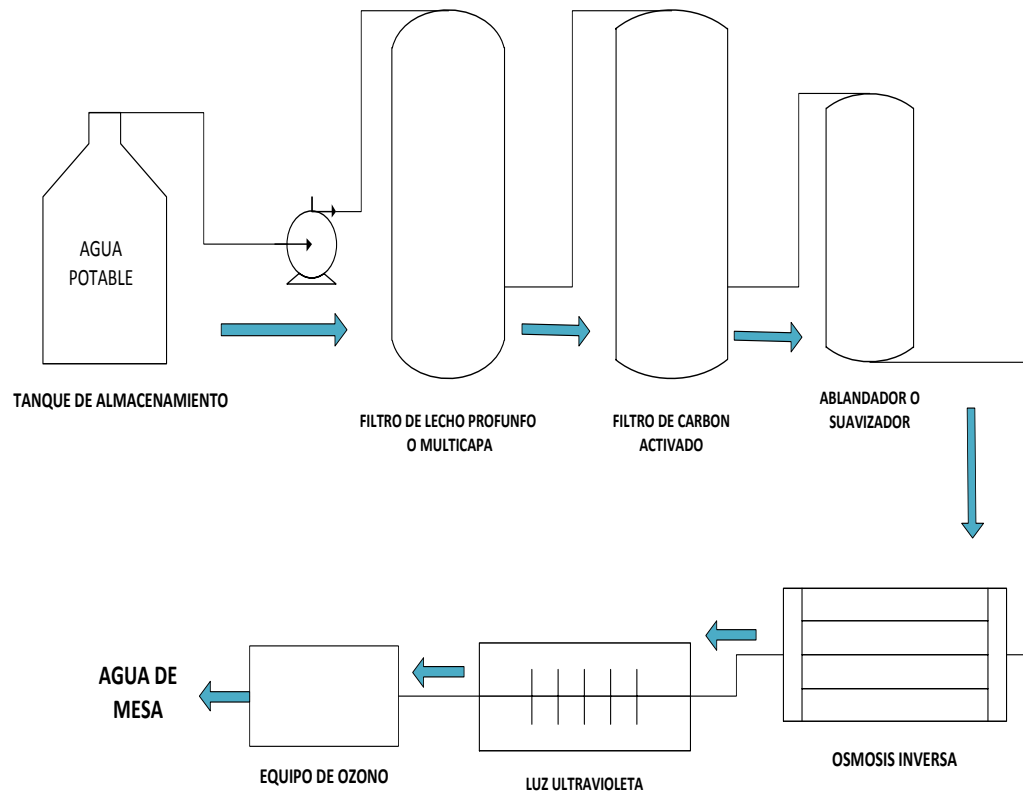
Figura 3-1: Diagrama de flujo con ósmosis inversa
