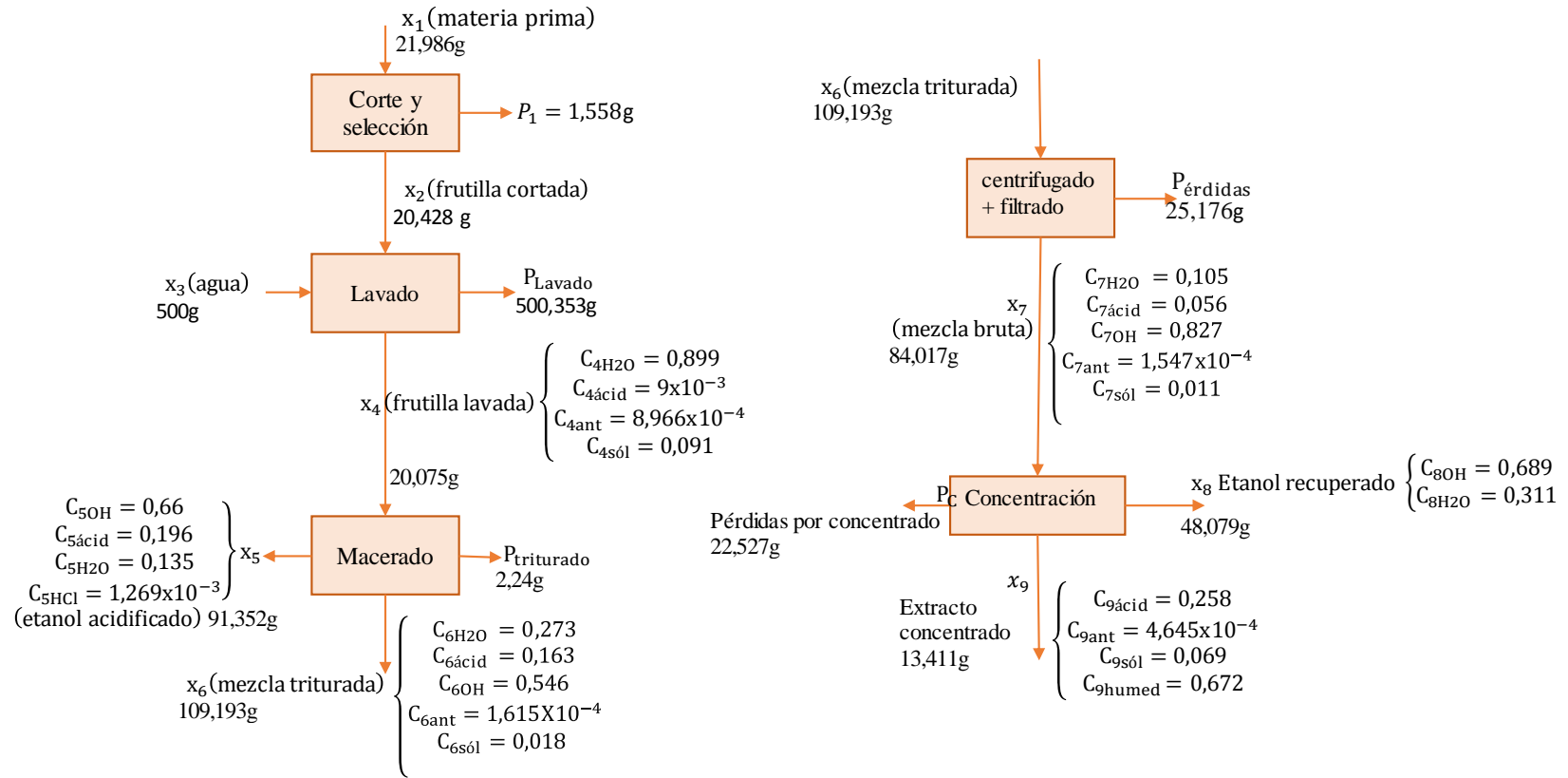
Ilustración IV-2 Esquema del balance de materia
