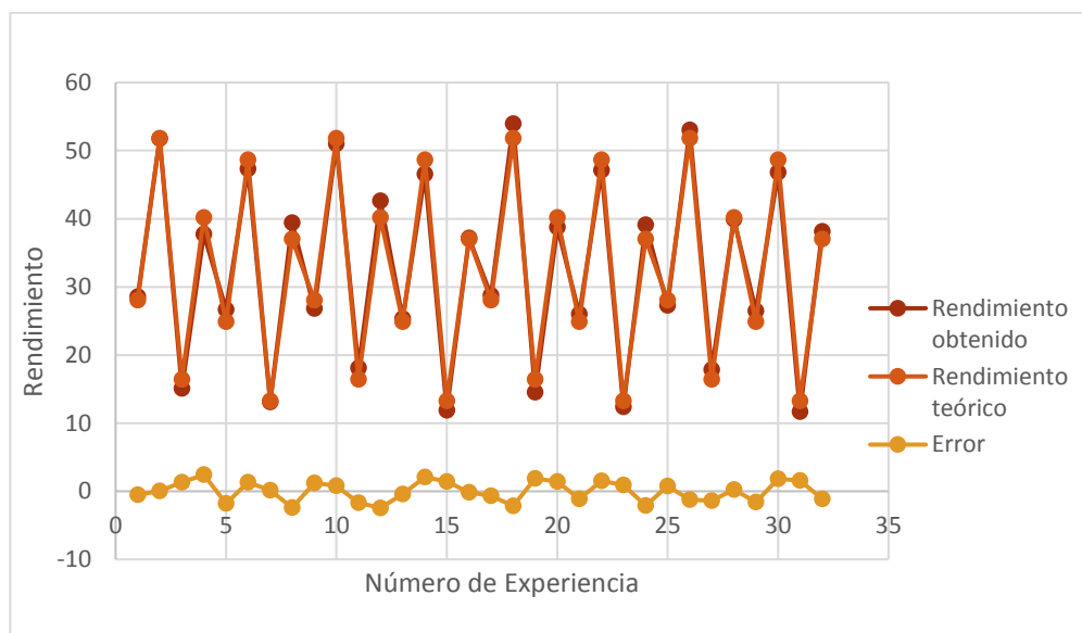
Ilustración V-0-8 Gráfica del rendimiento teórico, obtenido y error
