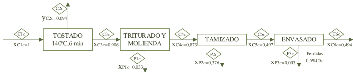
Figura 3-26 Diagrama de bloques – flujo general del proceso de obtención de harina pre cocida de cebada
