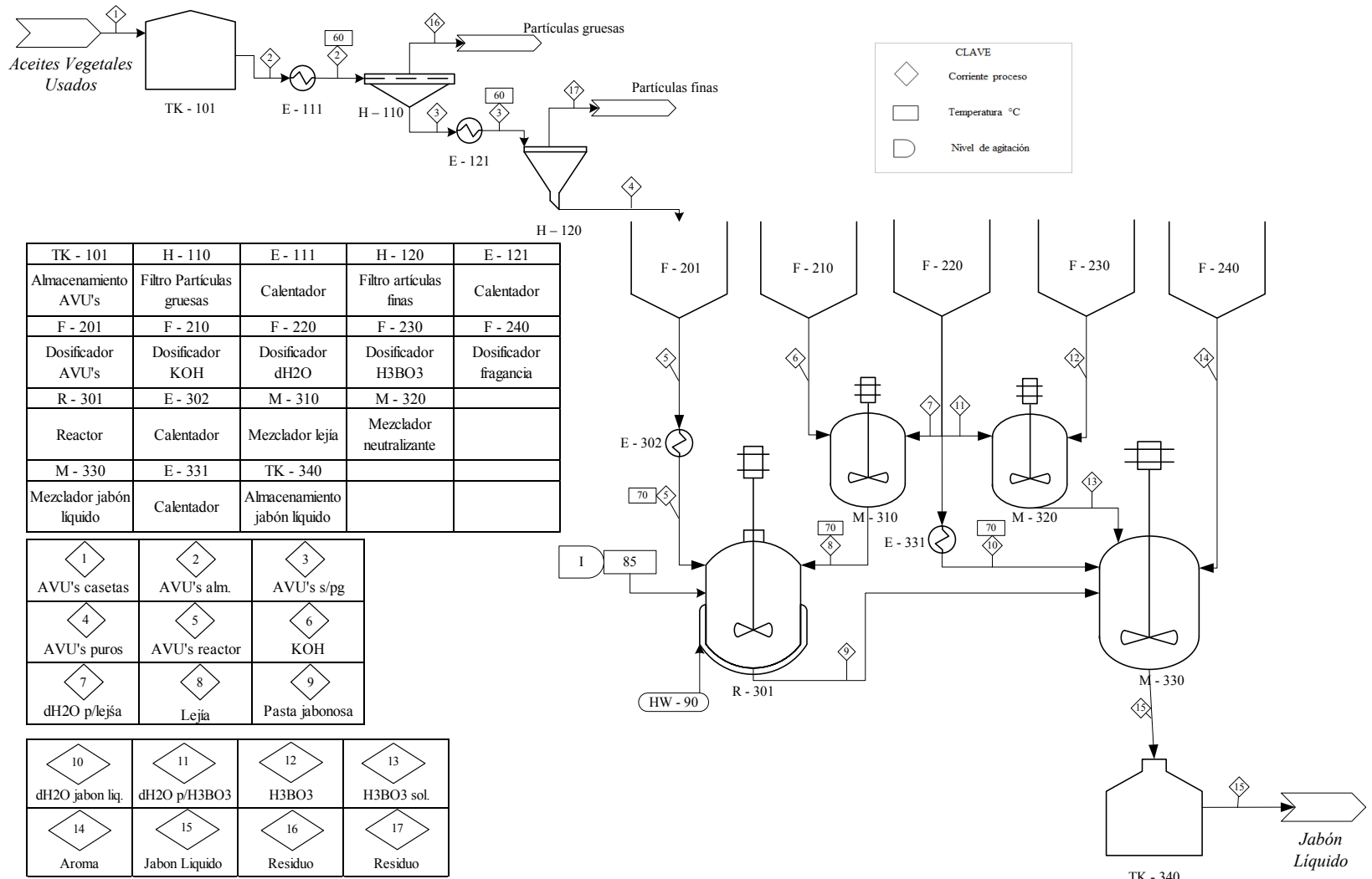
Figura 3-2 Diagrama PFD del proceso
