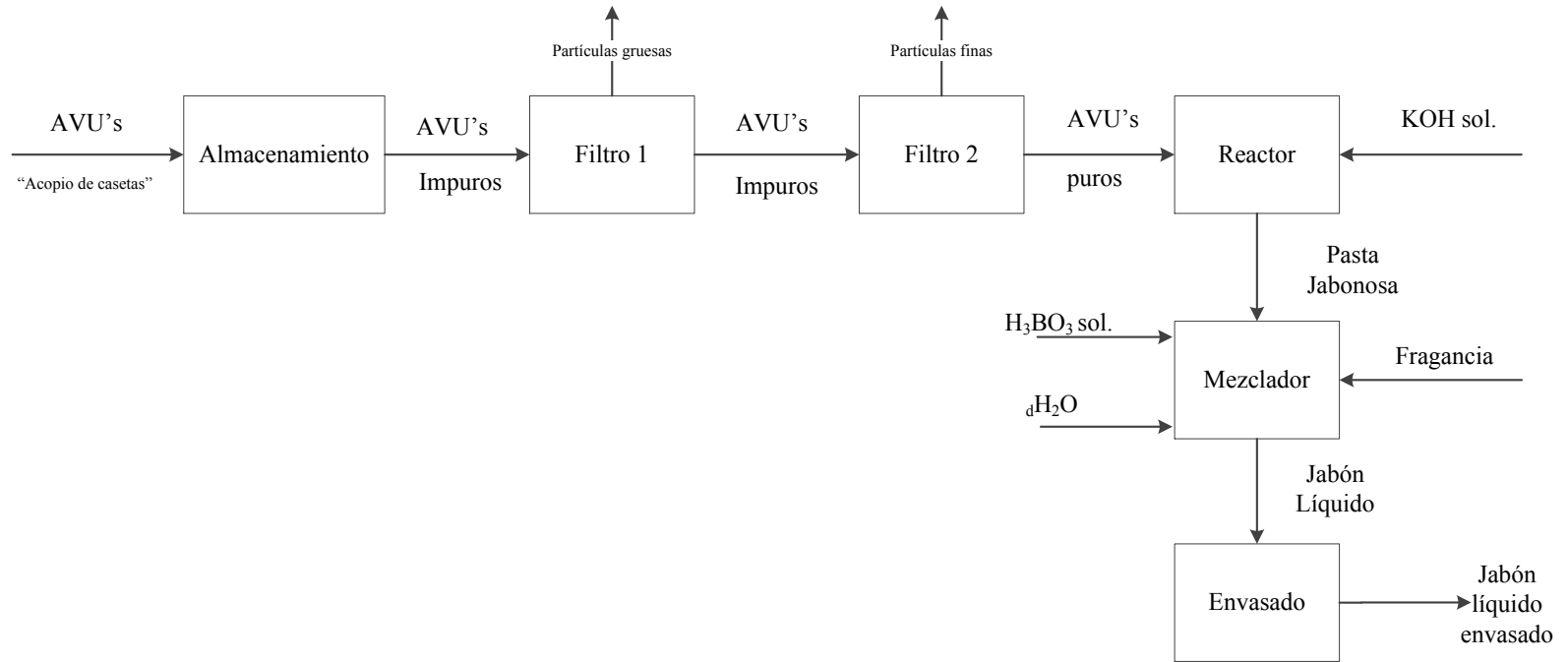
Figura 3-1 Diagrama de Bloques Elaboración de Jabón Líquido
