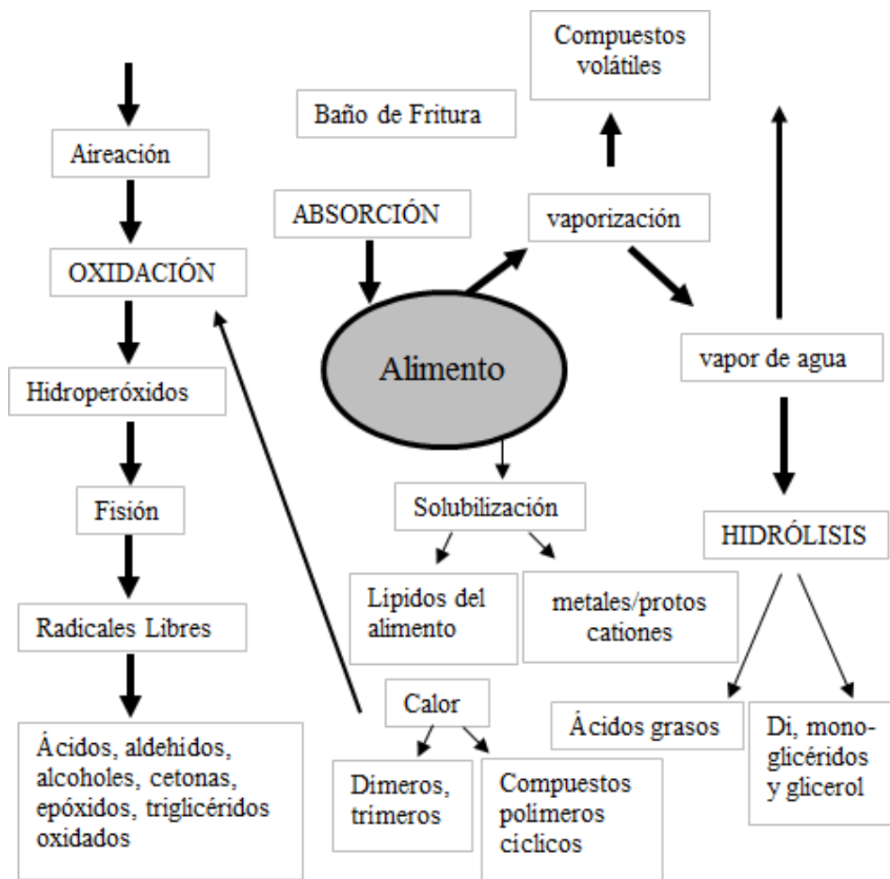
Figura 2-2 Reacciones Químicas en el Proceso de Fritura
