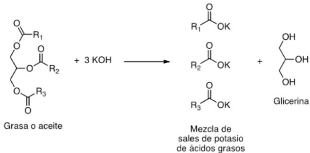
Figura 2-3 Saponificación
