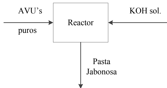
Figura 4-20 Diagrama de Bloques en el Reactor
