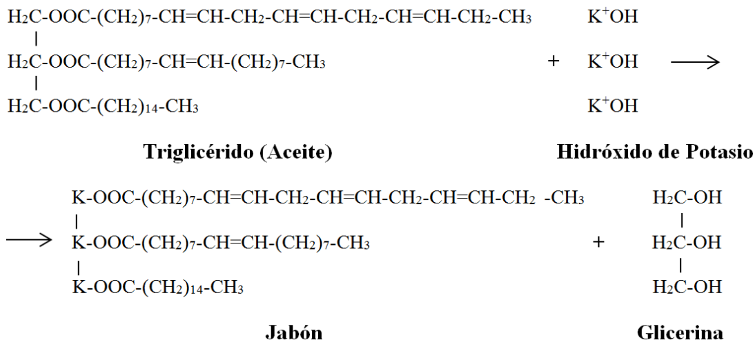
Figura 4-23 Reacción química de saponificación
