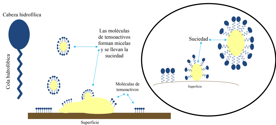
Figura 2-4 Mecanismo de Acción de los Tensioactivos.
