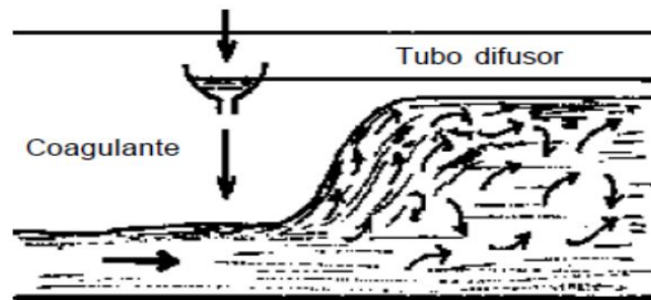
Figura III-6. Resalto hidráulico
