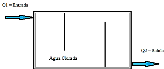
Figura III-12. Esquema de cámara de contacto
