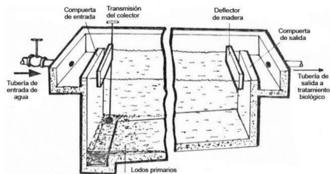
Figura III-3. Desarenador
