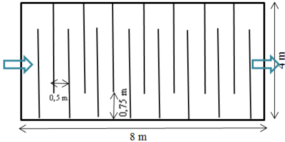
Figura 3-3. Vista en Planta del Humedal Artificial con sus respectivas dimensiones. Elaboración Propia
