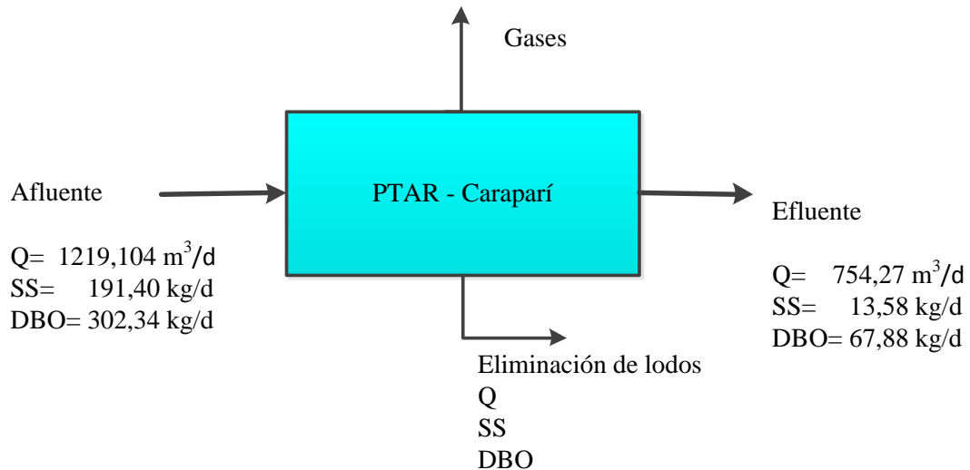
Figura 3-1. Diagrama para el Balance General de Materia. Elaboración Propia
