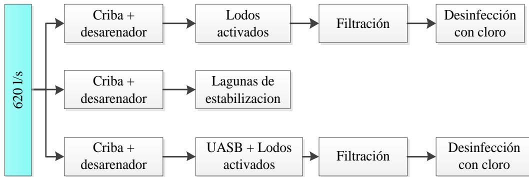
Figura 1-1. Configuración de Trenes de Tratamiento Representativos en Latinoamérica. Adaptado de Noyola, Morgan y Güereca (2013)
