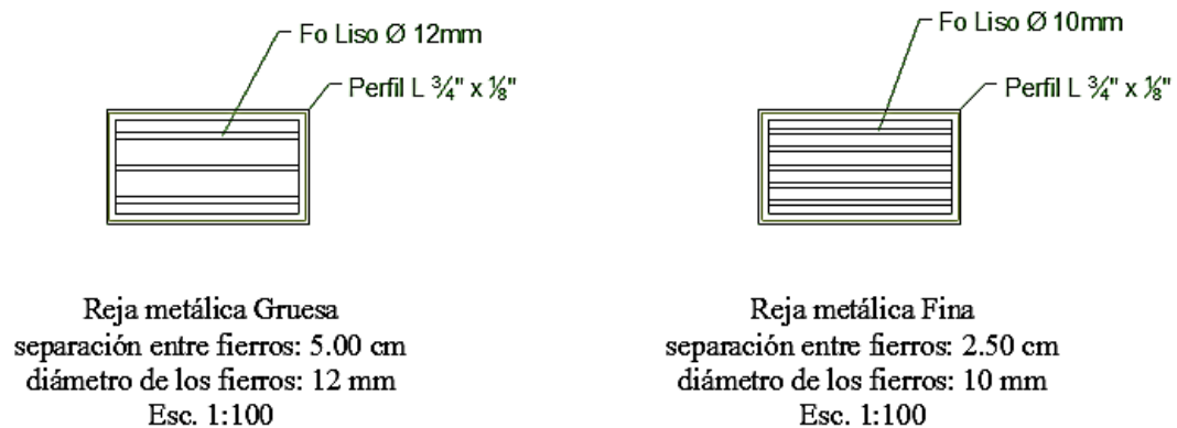
Figura 1-6. Plano de rejillas. Saneamiento básico del Gobierno Autónomo Municipal de Caraparí (2018)
