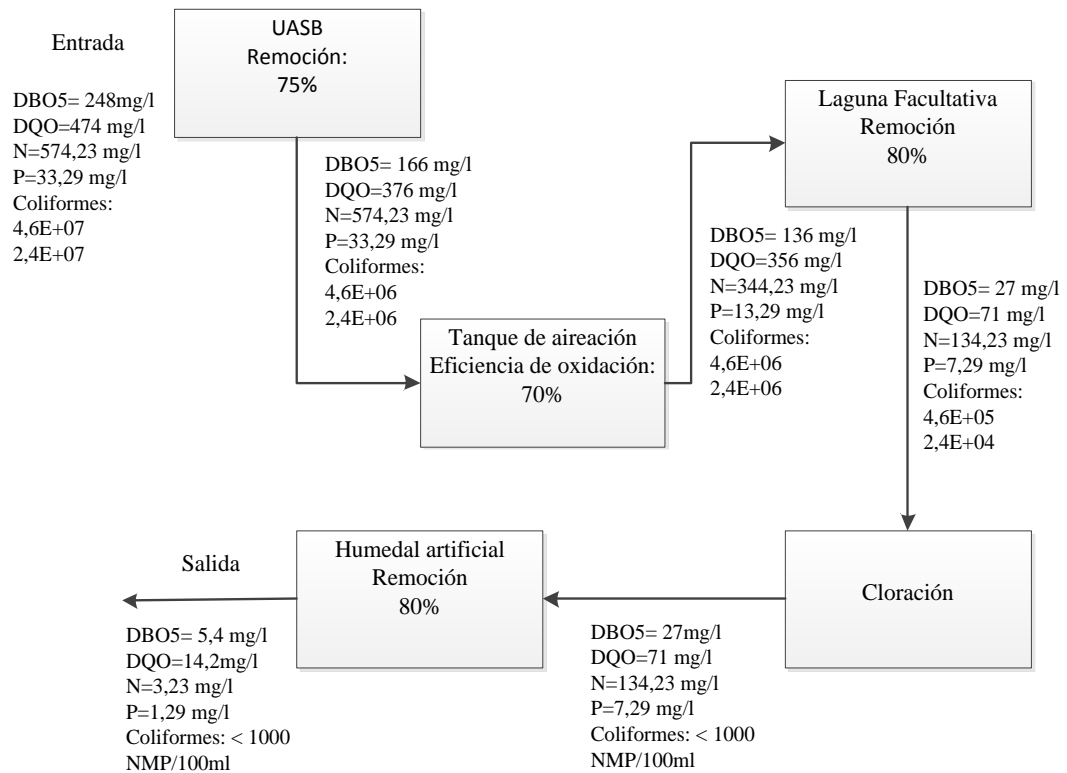
Figura 3-10. Eficiencia del Proceso Optimizado, Resultados de la Remoción y Eliminación de Contaminantes. Nota. Datos basados solamente en eficiencias, no son resultados experimentales. Elaboración Propia
