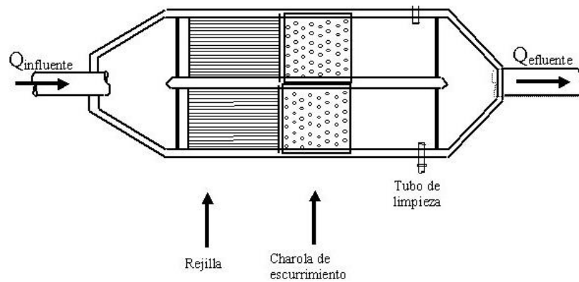
Figura 2-11. Vista en Planta de un Sistema Manual de Rejilla con dos Cámaras. (Henao, Salazar, & López, 2016)
