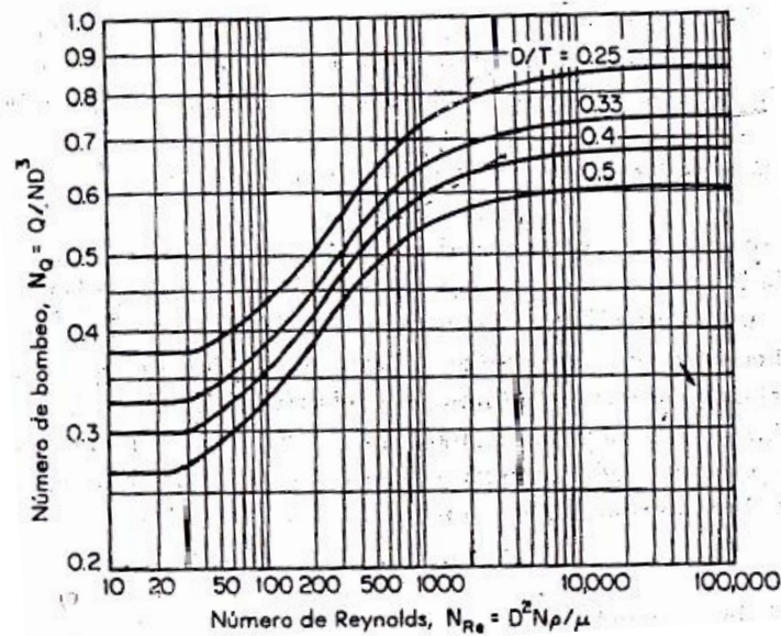
Figura 3-7. Numero de bombeo, en función del número de Reynolds del Impulsor, para impulsores con alabes inclinados ( N_p=1,37 ). Recuperado de Chohey (1988)
