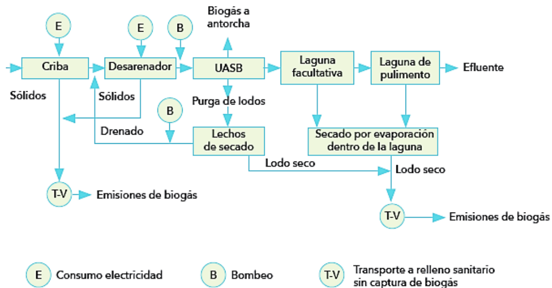
Figura 1-2. Diagrama de Flujo de UASB + Lagunas de Facultativa y de Pulimento. Noyola (2013).
