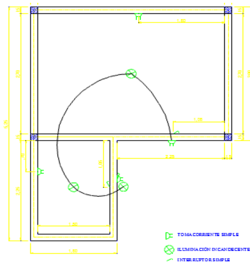
Figura 1-15. Plano Eléctrico. Saneamiento básico del Gobierno Autónomo Municipal de Caraparí (2018)
