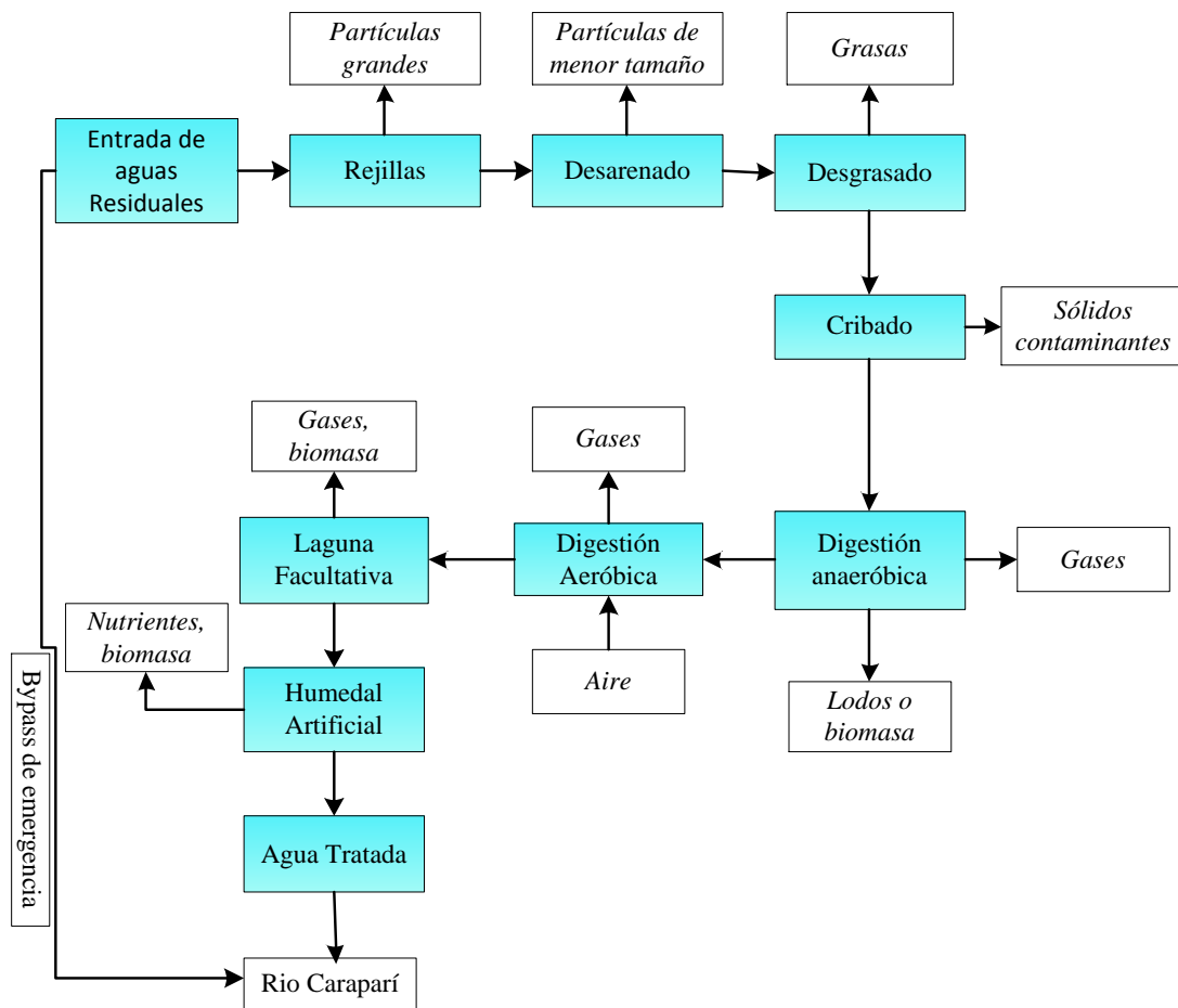
Figura 2-2. Diagrama de bloques del proceso actual de tratamiento de la Planta de Tratamiento Aguas Residuales de Caraparí. Elaboración propia
