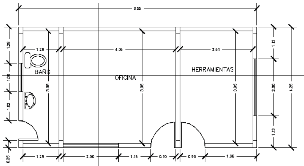
Figura 1-14. Plano de la caseta de controles. Saneamiento básico del Gobierno Autónomo Municipal de Caraparí (2018)
