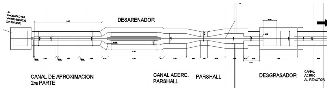
Figura 1-7. Plano del Desarenador, Canal Parshall y Desgrasador. Saneamiento básico del Gobierno Autónomo Municipal de Caraparí (2018)
