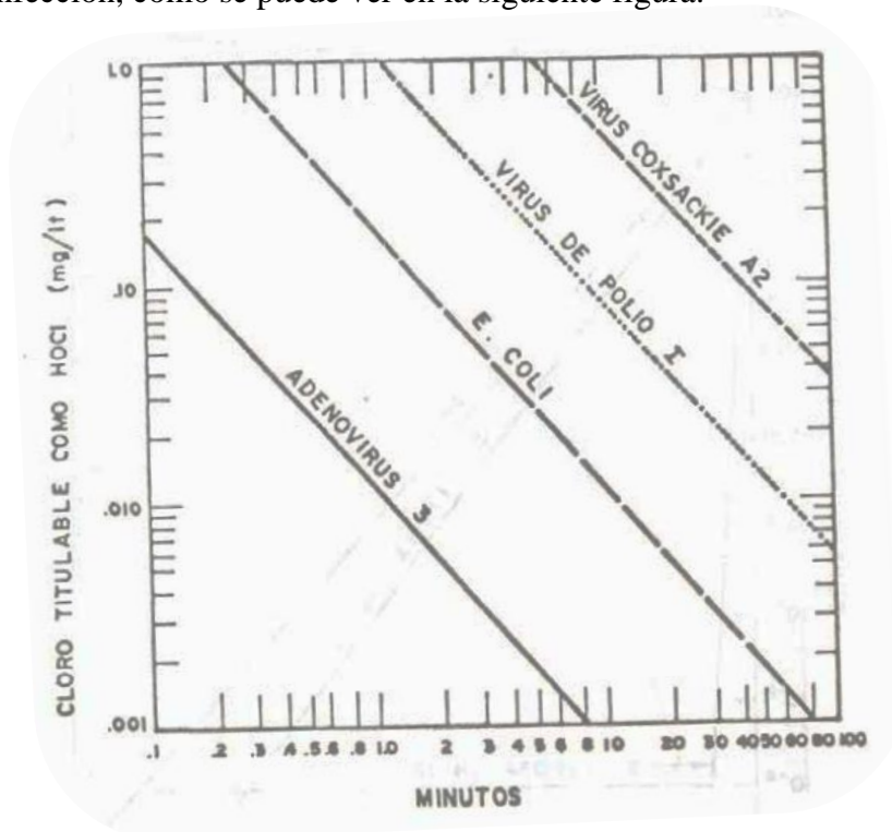
Figura 2-15. Relación entre Concentración y Tiempo en que el HOCL Destruye Diferentes m.o. Arboleda (2000)
