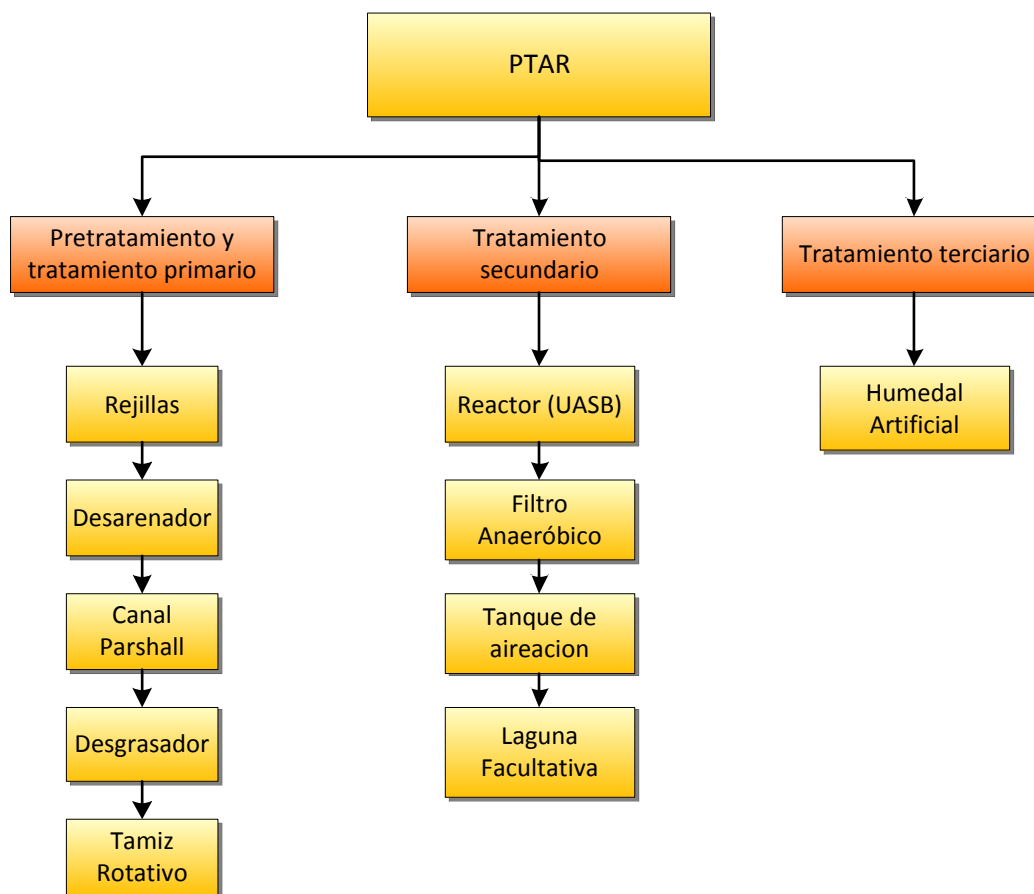
Figura 1-4. Diagrama de Bloques, Distribución de la PTAR de Caraparí. Elaboración propia
