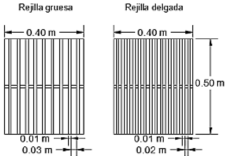
Figura 2-12. Dimensiones de las rejillas. Henao (2016)
