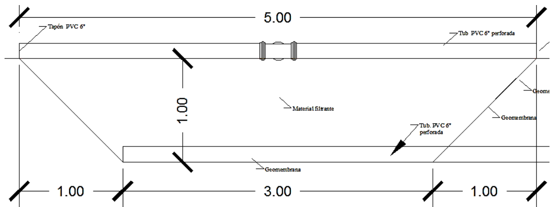
Figura 1-12. Corte Transversal del Humedal Artificial. Saneamiento básico del Gobierno Autónomo Municipal de Caraparí (2018)
