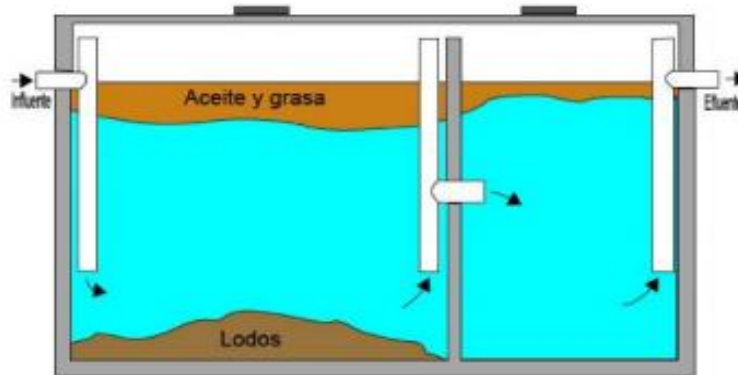
Figura 2-14. Vista Interna de una Trampa de Grasas
