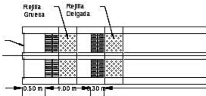
Figura 2-13. Vista en planta del desarenador y la ubicación de rejillas. Henao (2016)
