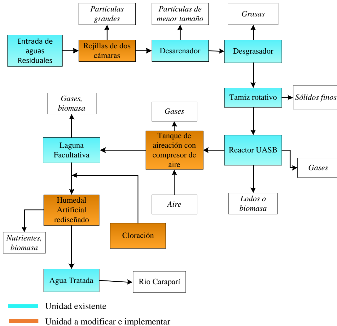
Figura 3-9. Diagrama de bloques del proceso optimizado. Elaboración Propia
