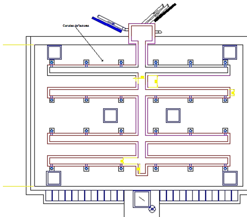
Figura 1-8. Planta Superior del Reactor UASB. Saneamiento Básico del Gobierno Autónomo Municipal de Caraparí (2018)
