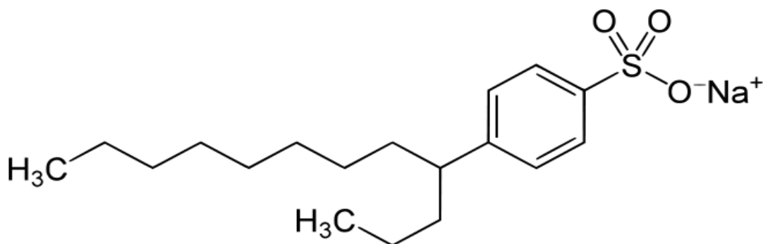
Alkil – Aril sulfonato de sodio
