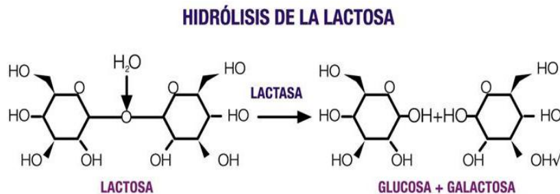
Figura 3-3: Reacción Enzimática de la Lactasa
