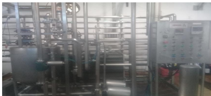
Figura 3-20: Pasteurizador por Placas de PIL Tarija S.A.
