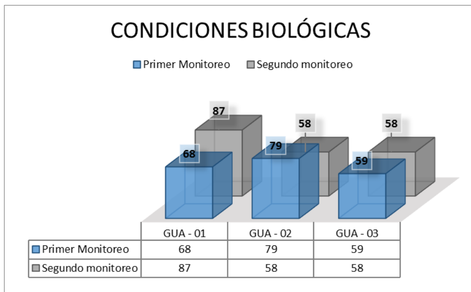
Gráfico 12. Variación de Condiciones Biológicas en los puntos de muestreo del río Guadalquivir
