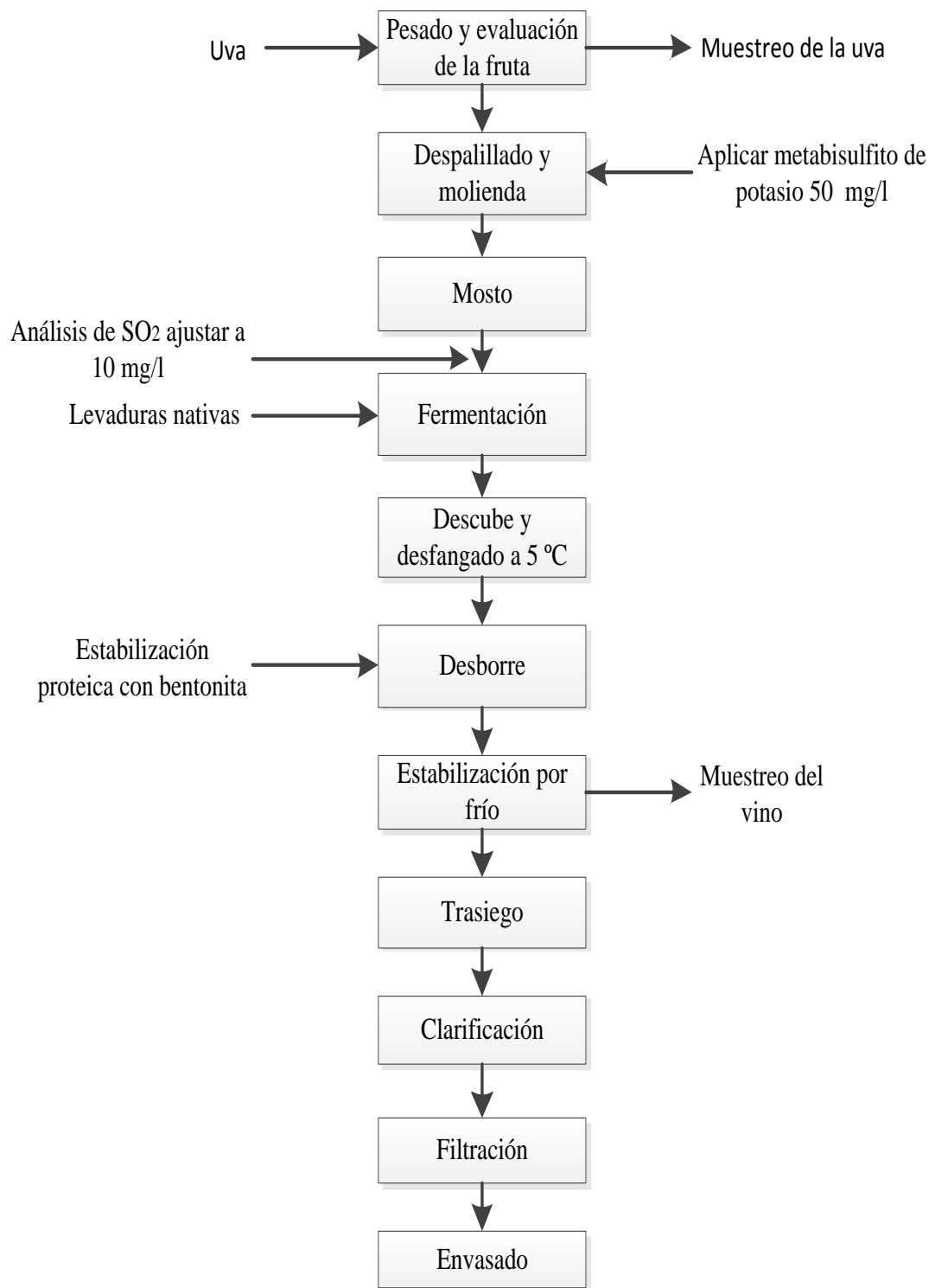
Figura 3-4. Diagrama de bloques del vino blanco descubado en (tf)
