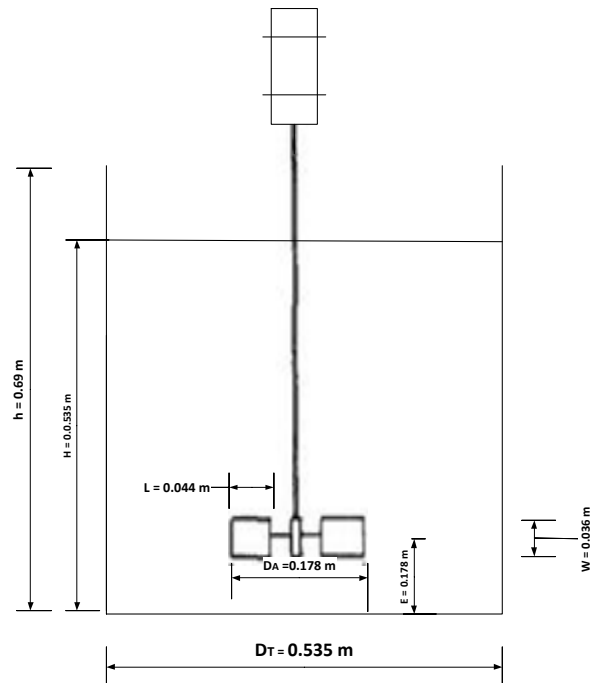
Figura II – 31: PLANO DEL TANQUE CON AGITADOR
