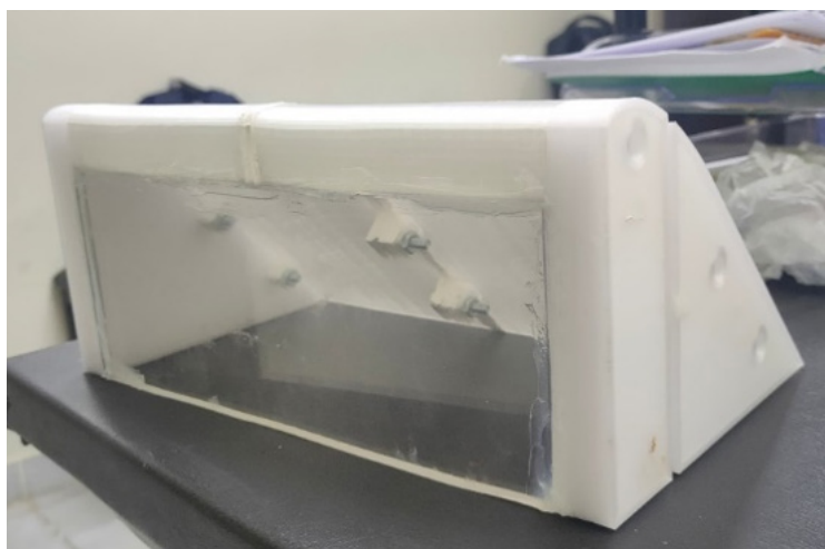
Vertedero tipo Creager de 30 cm de longitud
