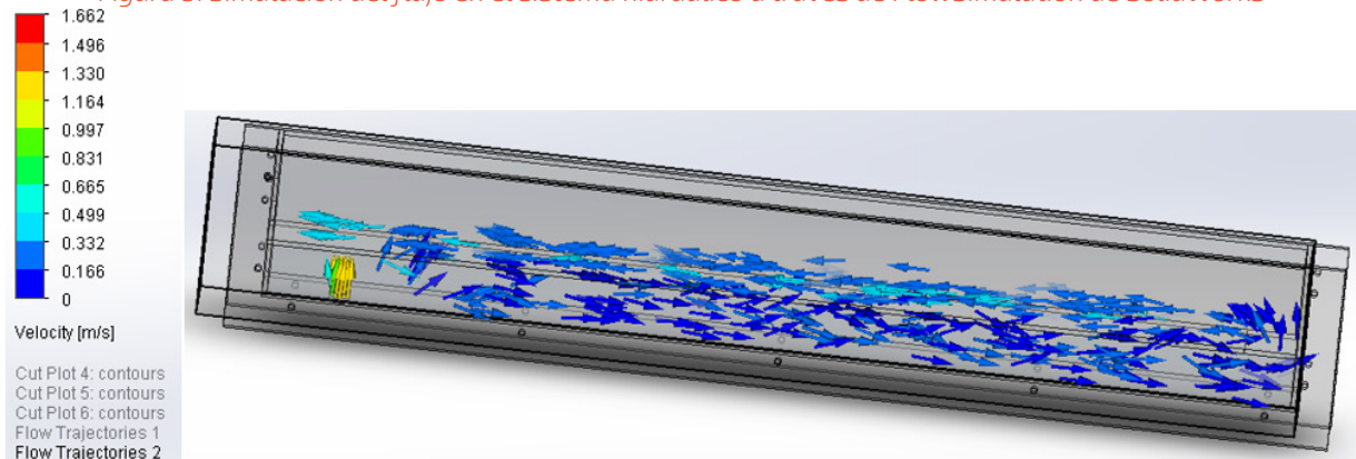
Simulación del flujo en el canal de vidrio para un caudal mínimo de 10 litros/minuto
