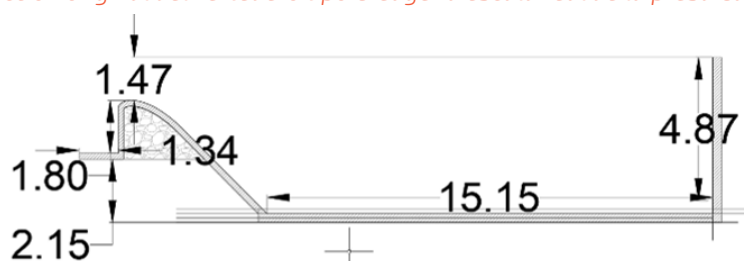
Figura 3: Sección original del vertedero tipo Creager a escala real de la presa Carachimayo
