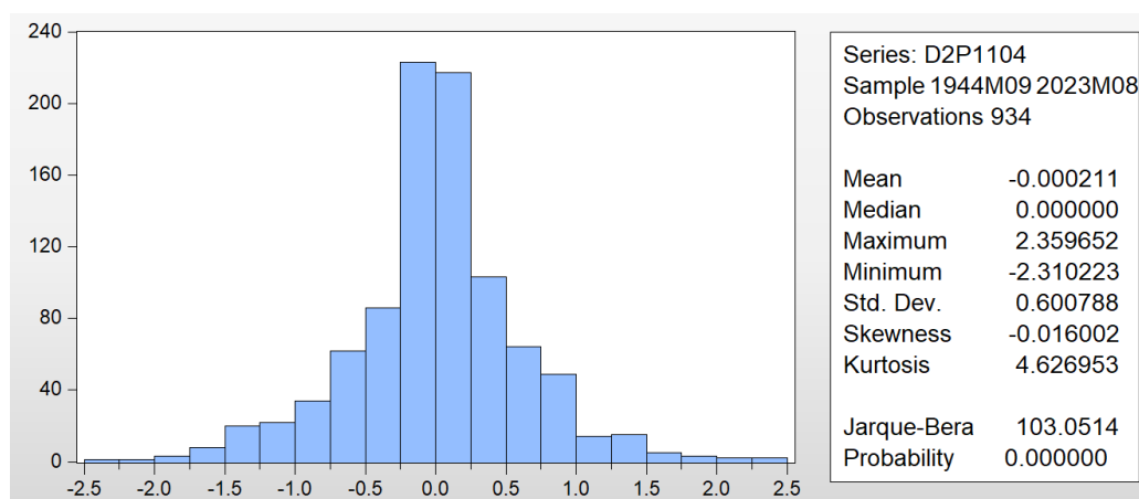
Figura 6: Modelo Arima (0,2,2)/Sarima (1,1,1) para la serie temporal de precipitación media mensual diferenciada en 2 y 12 pasos, graficas FAP y FAC y distribución gaussiana de errores. Estación Tarija AASANA Precipitación mensual estación AASANA Tarija
